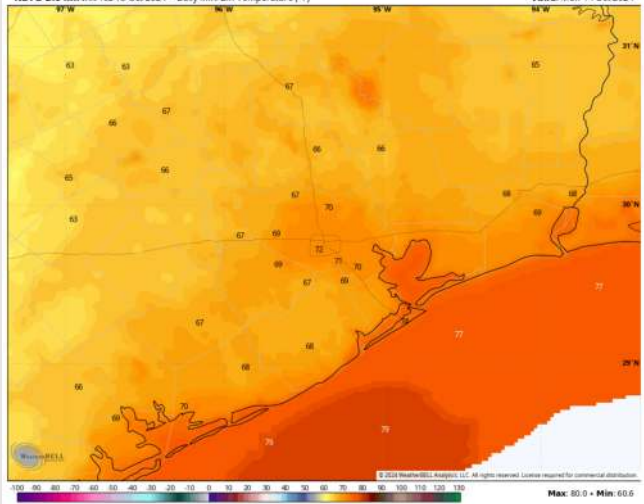
NDFD 2.5 km Init 16z 13 Oct 2024 • Daily Min 2m Temperature (°F) Valid: Mon 14 Oct 2024
